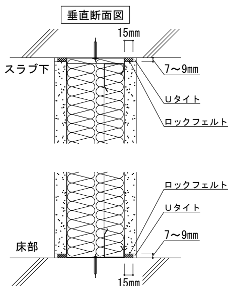
<スラブ下および床部の納まり例>
